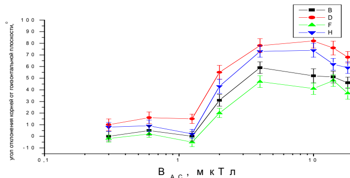
Рис. Зависимости угла отклонения от горизонтальной плоскости при частоте переменной составляющей f=6.85 \text{ Гц} от амплитуды переменной составляющей магнитного поля. Кривая F соответствует времени 0.5 часа, B - 1 часу, H - 1.5 часам, D - 2 часам.
