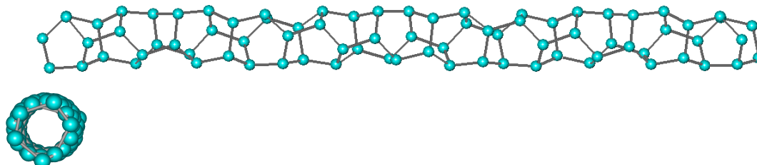
Рис.1. Кислородный аркас жидкокристаллической структуры воды для спирали 30/11.
