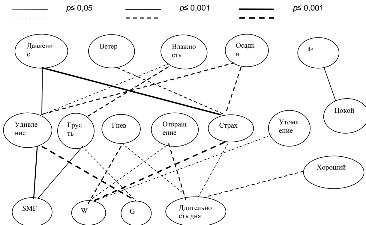
Рис.1. Корреляционные плеяды по средним для каждого из 12 имен за 12 дней с 1.2. по 5.4. 2013.
