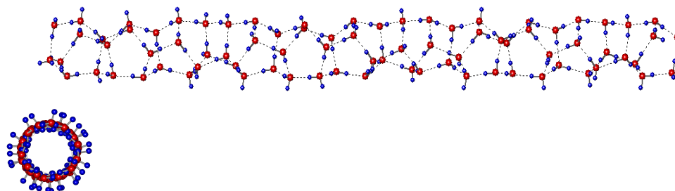
Рис.2. Та же структура для спирали 30/11 с расположением протонов.
