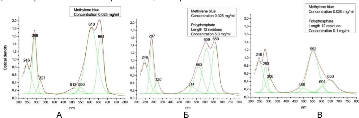
Рис. 1. Спектры поглощения растворов метиленового синего и его комплексов с полифосфатом натрия (длина ПФ-цепи 16-18) разной концентрации (А - концентрация полифосфата 0 мг/мл, цвет раствора плотно синий; Б - концентрация полифосфата 5 мг/мл,
