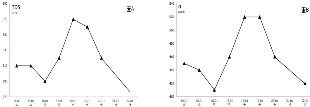
Рис. 1 Изменения параметров \sigma и TDS воды «Ордана»
