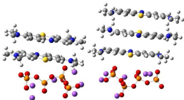
Рис. 2. Компьютерное моделирование ассоциатов метиленового синего при их взаимодействии с тетрафосфатом.
