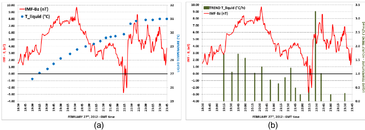
Рис. 2 Всплеск температуры воды (а) и скорости нагрева (б) в течение 10-15 минут после двойной инверсии B_z компоненты межпланетного магнитного поля 27 февраля 2012 года.
