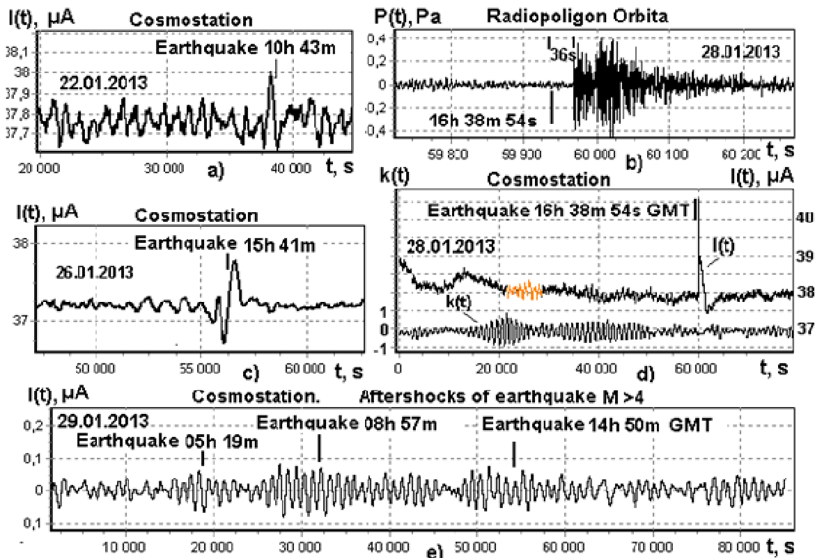
Рисунок 1 - Вариации тока I(t) в ЭВЯ 22.01.2013 - (а); Инфразвуковой сигнал от землетрясения M=6,1 - (b); Вариации тока в ЭВЯ 26.01.2013 - (с); Вариации тока в ЭВЯ и результат расчета автокорреляционной функции k(t) в дни землетрясения 28.01.2013 - (d) и афтершоков 29.01.2013 - (е). По оси X - время от начала суток по времени GMT в секундах.
