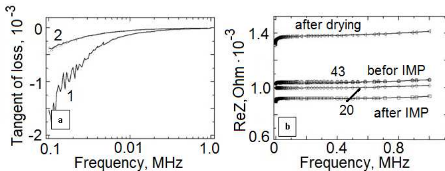
Рис. 1. Зависимость \text{tg}(\delta) (a) и \text{Re}Z (b) от частоты до (1) и после (2) ИМП — воздействия. Числа на рис 2b указывают время измерения в часах после магнитоимпульсного воздействия Fig. 1. Dependence of \text{tg}(\delta) (a) and \text{Re}Z (b) on frequency before (1) and after (2) PMF; 2b -The numbers indicate measurement time in hours after magnetic pulse influence
