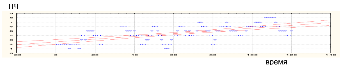
Рис. 2. Зависимость ПЧ (объяснение в тексте) от времени (сутки) с 4.12.12 по 2.04.13.
