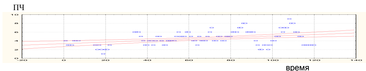
Рис. 1. Зависимость ПЧ (объяснение в тексте) от времени (сутки) с 4.12.11 по 1.04.12.
