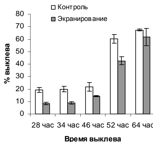
Рис. 2. Действие экранирования на динамику выклева науплиев из цист артемии
