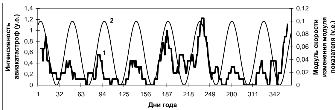
Рис. 1. Сопоставление распределения интенсивности авиакатастроф (кривая 1) и вариаций модуля скорости изменения модуля показателя (отклонения СВЗ или нутации, кривая 2) в течение года
