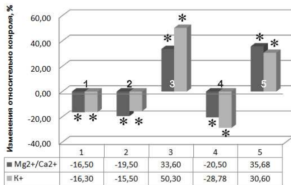
Рис. Изменение Mg^{2+}/Ca^{2+} - и K^+ -АТФ-азной активности (%) во времени под действием ЭМП КНЧ ( n=50 ). * - достоверные различия относительно значений без воздействия ЭМП, p < 0,05 .
