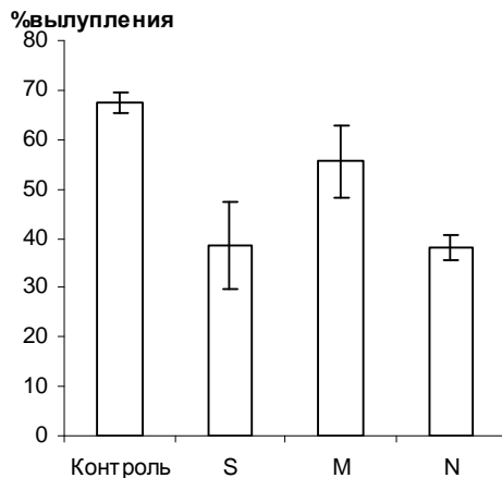
Рис. 1. Действие постоянного магнитного поля на выклев артемии ( S – южный полюс, M – середина, N – северный полюс)
