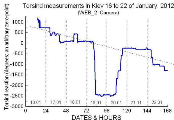
Рис. 2. Изменение отсчетов торсинда в период с 16 по 22 января 2012.
